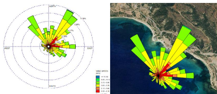
Figuras 39 y 40. Rosa de viento con su índice y representación de la rosa de viento sobrepuesta en la ubicación de la boya oceanográfica SPOT-30318R, correspondiente a la boya de Punta Arena, en la estación climática húmeda, entre junio y noviembre.
