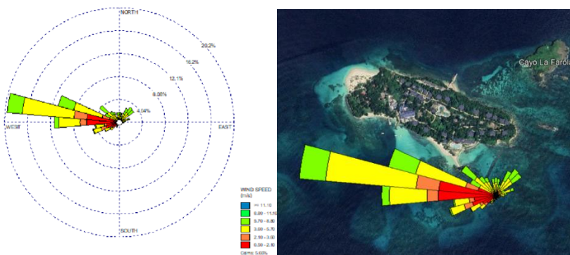
Figuras 21 y 22. Rosa de viento con su índice y representación de la rosa de viento sobrepuesta en la ubicación de la boya oceanográfica SPOT-30314R, correspondiente a la boya de Samaná, en la estación climática húmeda, entre junio y noviembre.
