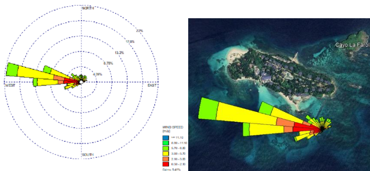
Figuras 19 y 20. Rosa de viento con su índice y representación de la rosa de viento sobrepuesta en la ubicación de la boya oceanográfica SPOT-30314R, correspondiente a la boya de Samaná, en la estación climática seca, entre diciembre y mayo.
